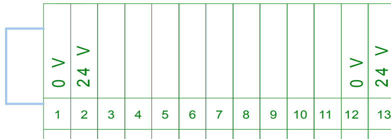
BORNIER DE COMMANDE VERT AIRCONTROL n°2
