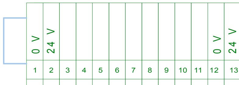
BORNIER DE COMMANDE VERT AIRCONTROL n°1
