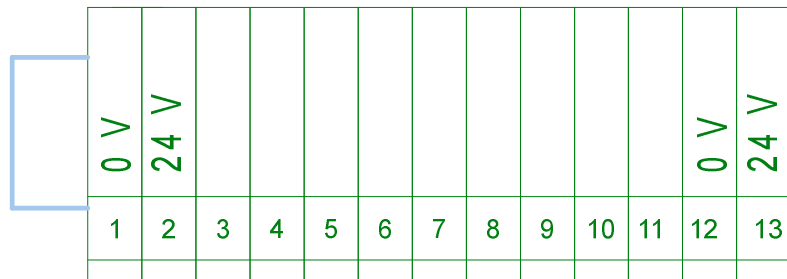
BORNIER DE COMMANDE VERT AIRCONTROL n°3
